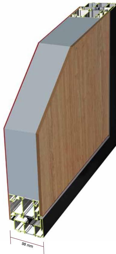
SISTEMA KORUS DOORS con rivestimento interno in legno
