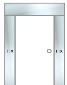
Porta ad una anta con sopra luce e fianchi luce
